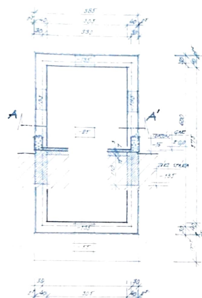
ZÁKLADY
