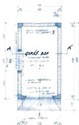
PŮDORYS
