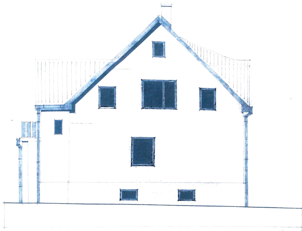
POHLED BOČNÍ :
